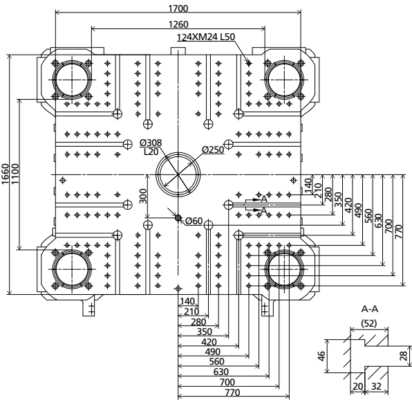
Fixed platen
